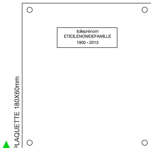
▲ NUMEROTATION : Petite plaquette inox avec inscription en noir 01
